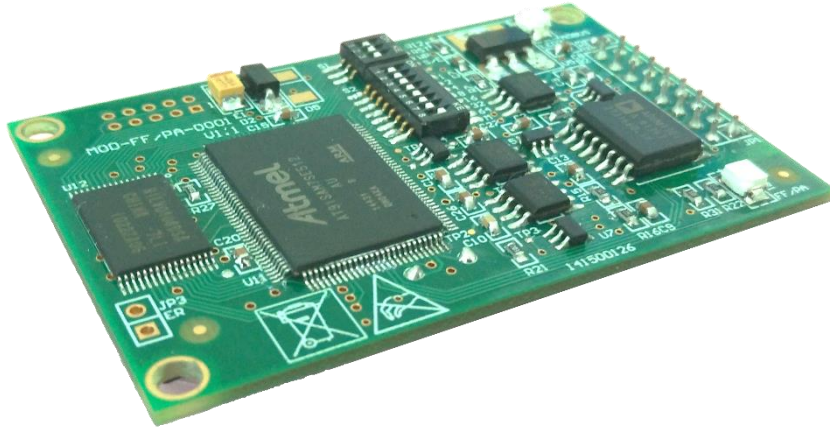
图 1.1 M0307 Modbus 转 PA 嵌入式模块
