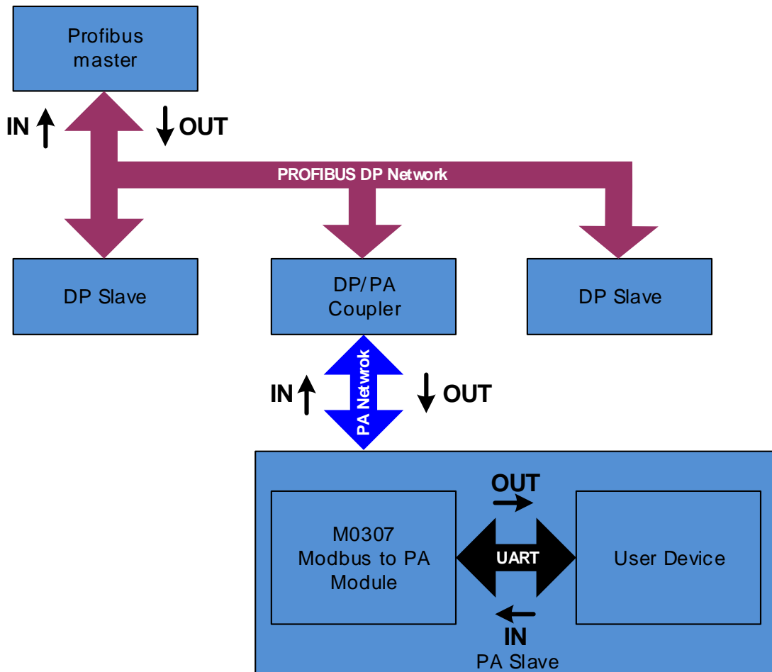
图 3.1 系统连接图
