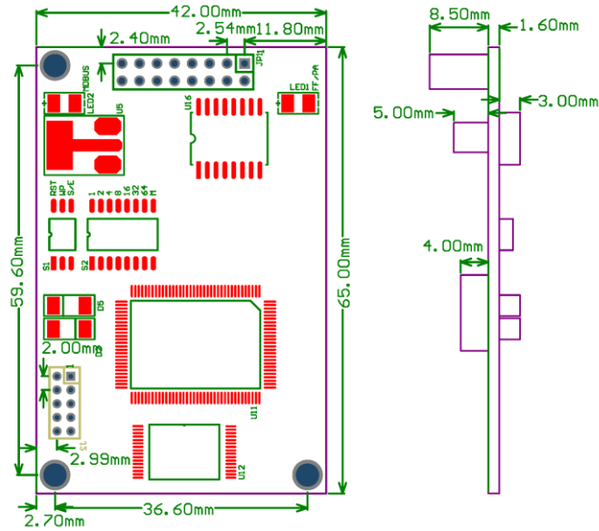
图 1.2 嵌入式模块设备外形尺寸（单位：mm）
