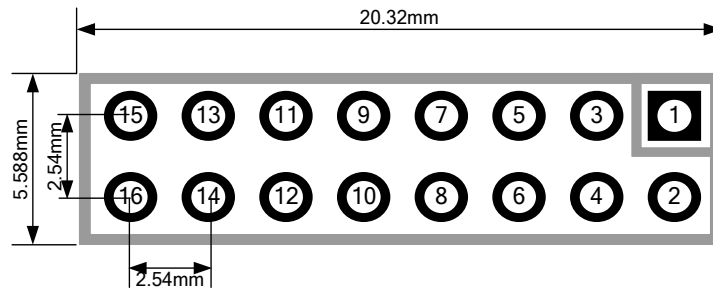
图 2.2 用户接口管脚定义及外型尺寸
