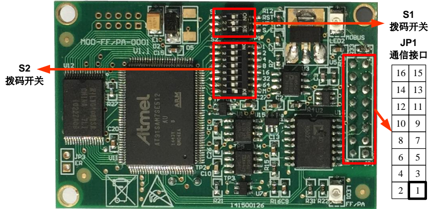
图 2.1 通信接口定义
