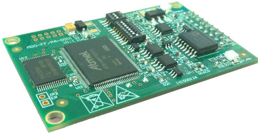
图 1.1 M0313 Modbus 转 FF 嵌入式模块
