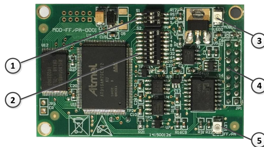
图 1.3 嵌入式模块结构
