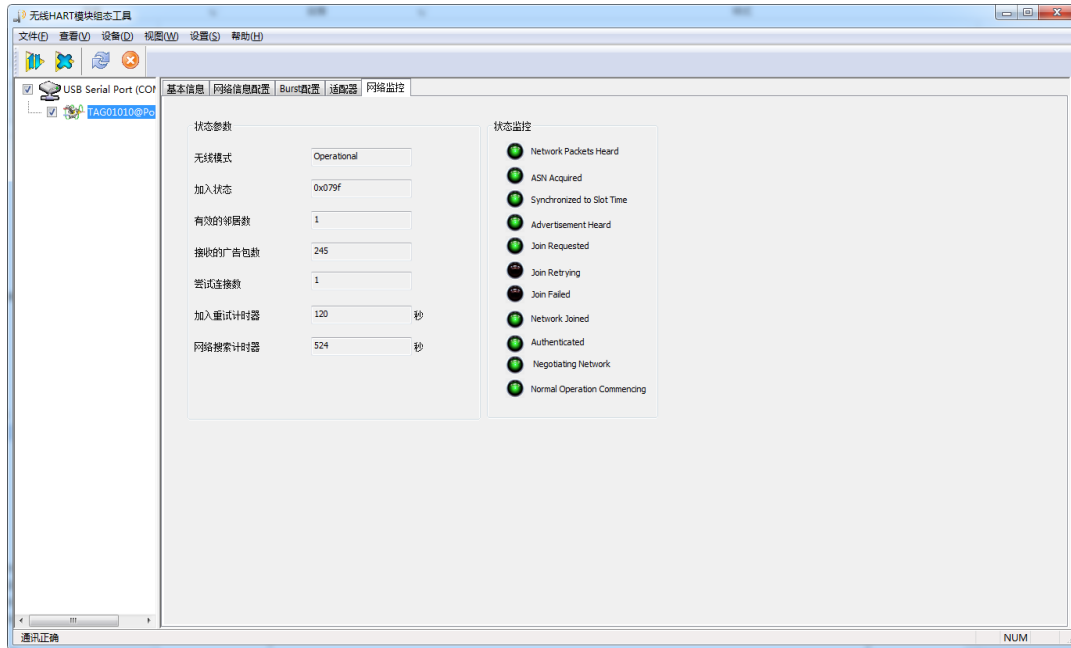
图 2-6 WirelessHARTMPT 组态软件网络监控界面
